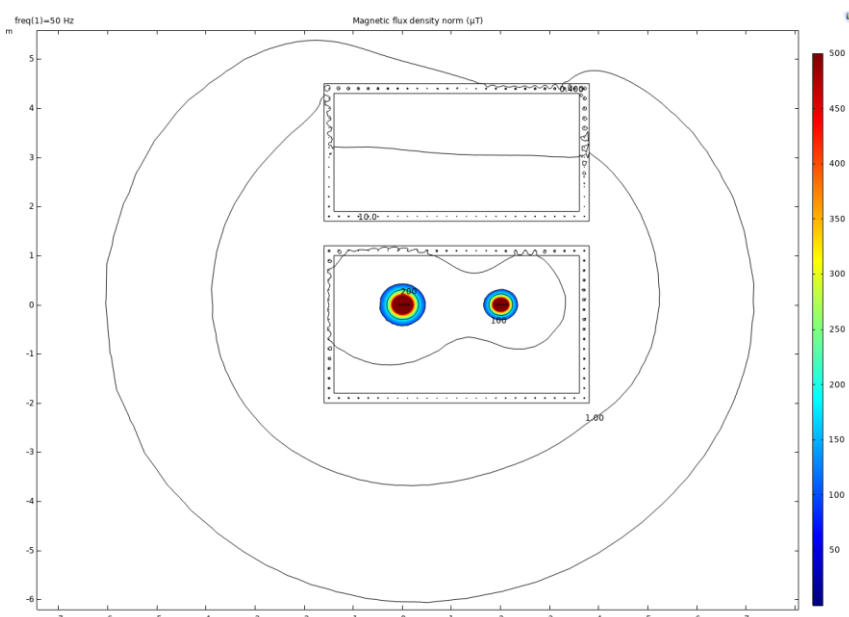
Figur 6 viser snitt av magnetfeltet i arealet over nettstasjonen uten skjerming. Magnetfeltet er sterkest nær nettstasjonen og avtar med økende avstand. Konturene viser avstanden som kreves for å være under utredningsnivået på 0,4 \mu\text{T} .
