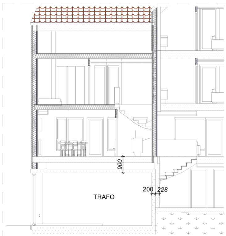
Figur 3: Snitt som viser transformatorrommets plassering i bygget og tilhørende arealer over og ved siden av transformatorene.
