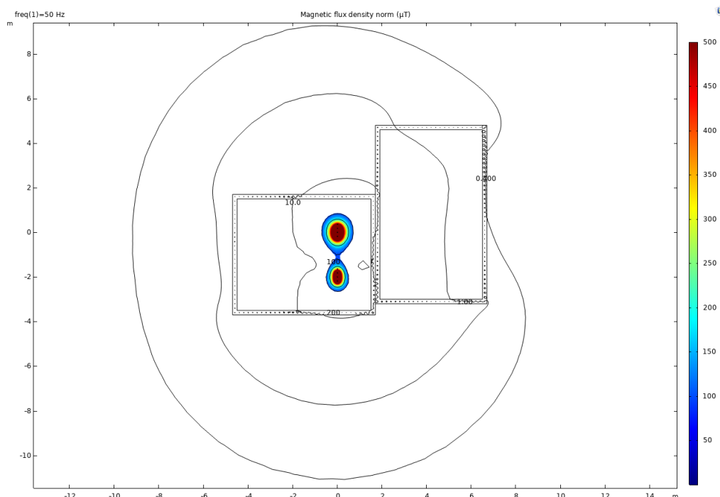
Figur 4 viser resultat av magnetfeltstyrke fra lavspentsiden uten skjerming. Magnetfeltet er sterkest nær lavspentsiden og avtar med økende avstand. Konturene viser avstanden som kreves for å være under utredningsnivået på 0.4 \mu\text{T} .
