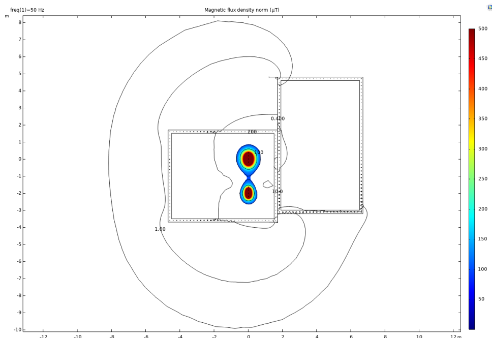
Figur 5 viser magnetfeltstyrken fra lavspentsidene med skjerming bestående av en 3 mm aluminiumsplate montert i vegg mellom nettstasjonen og tilstøtende arealer, samt tilhørende sideplater.
