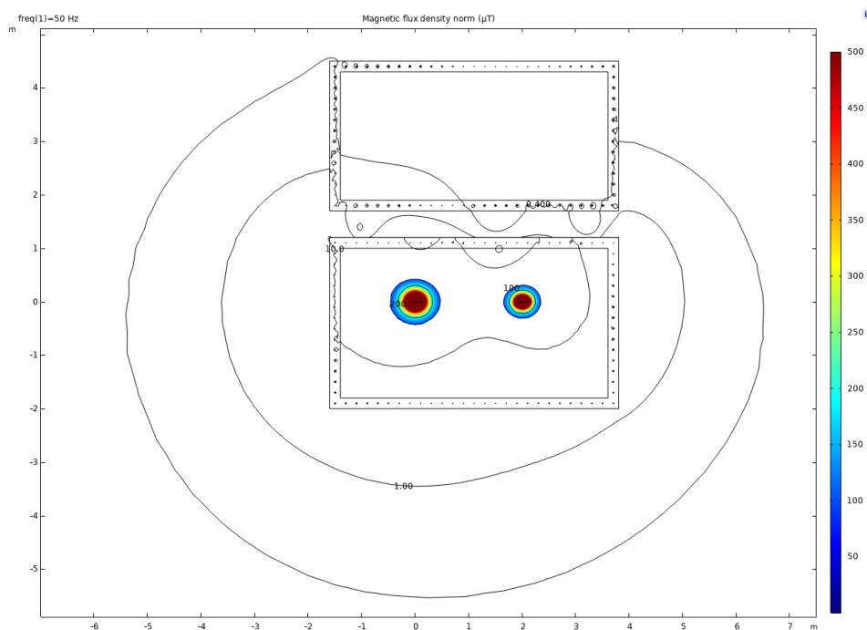
Figur 7 viser magnetfeltstyrken fra lavspentsidene med skjerming bestående av en 1 mm aluminiumsplate montert over taket til nettstasjonen.
