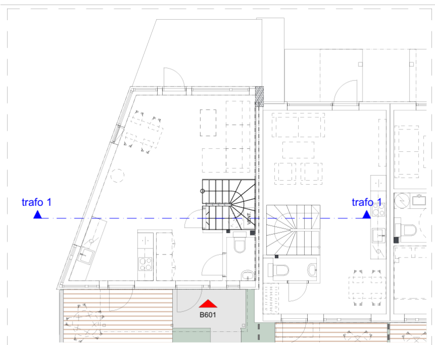
Figur 2: Planløsning av etasjen over transformatorrommet.
