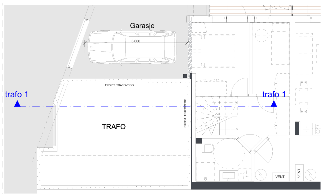
Figur 1: Planløsning av nederste etasje med plassering av transformatorrommet.
