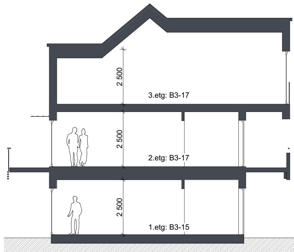
Snitt B3-15 og B-17
