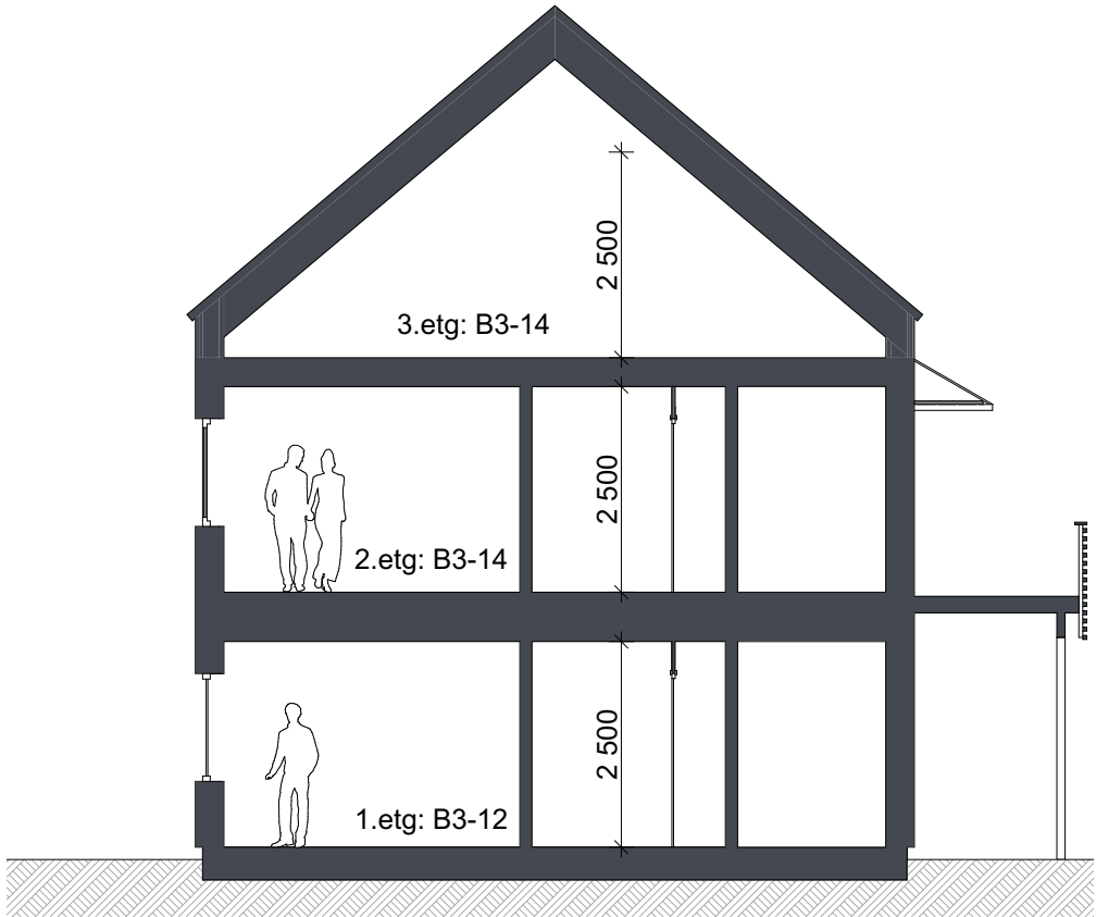
Snitt B3-12 og B-14
