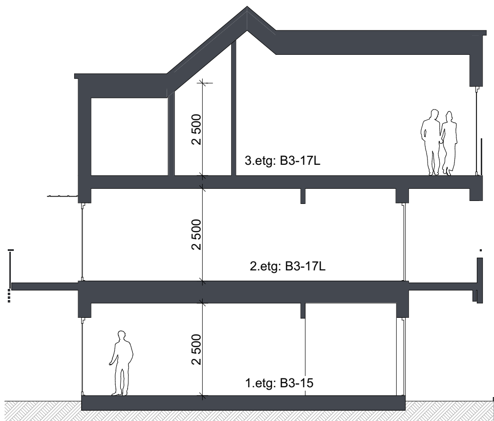
Snitt B3-15 og B-17L (innredet 3.etg)
