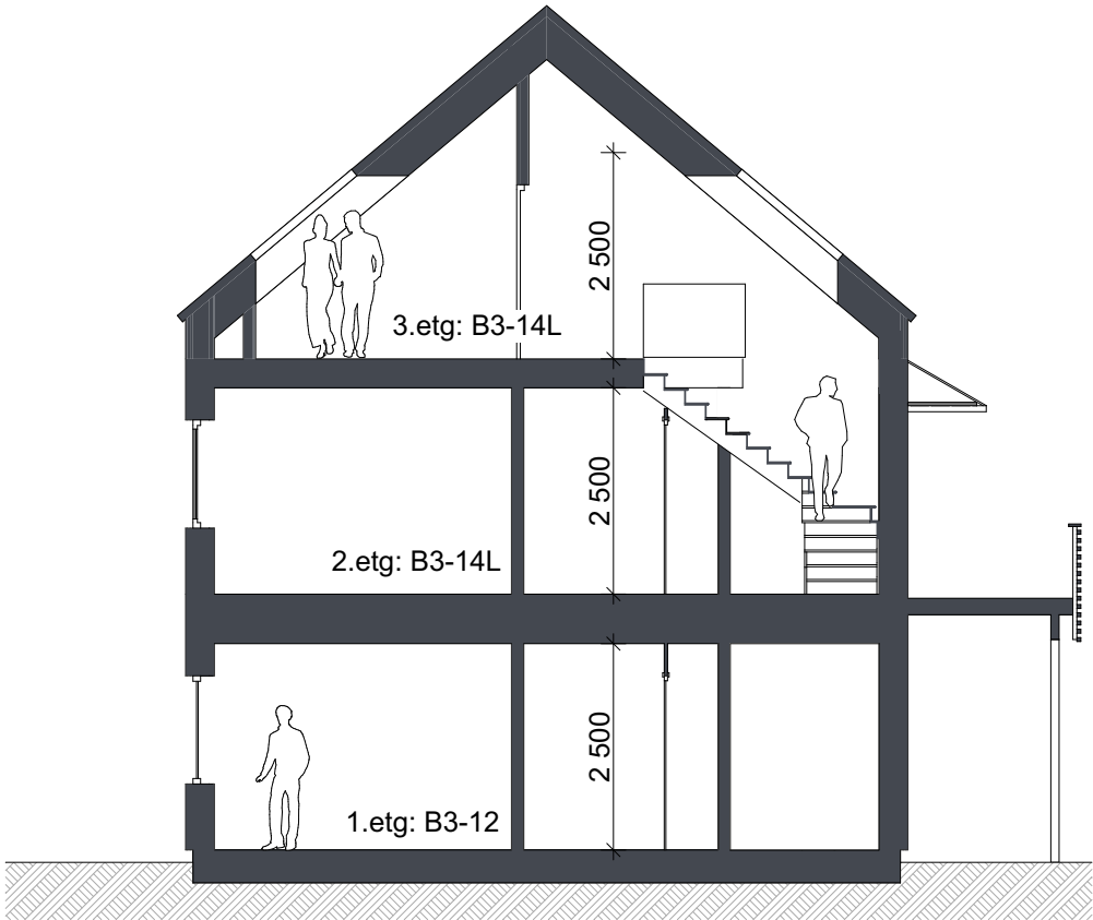
Snitt B3-12 og B3-14L (innredet 3.etg)
