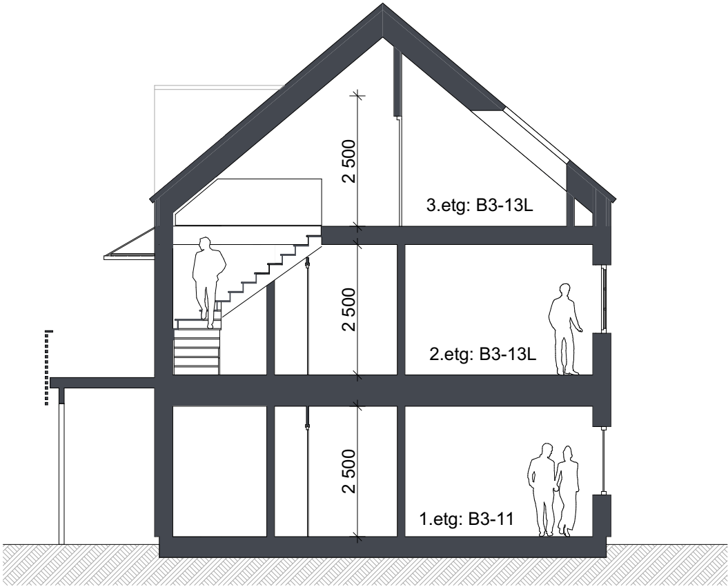
Snitt B3-11 og B3-13L (innredet 3.etg)
