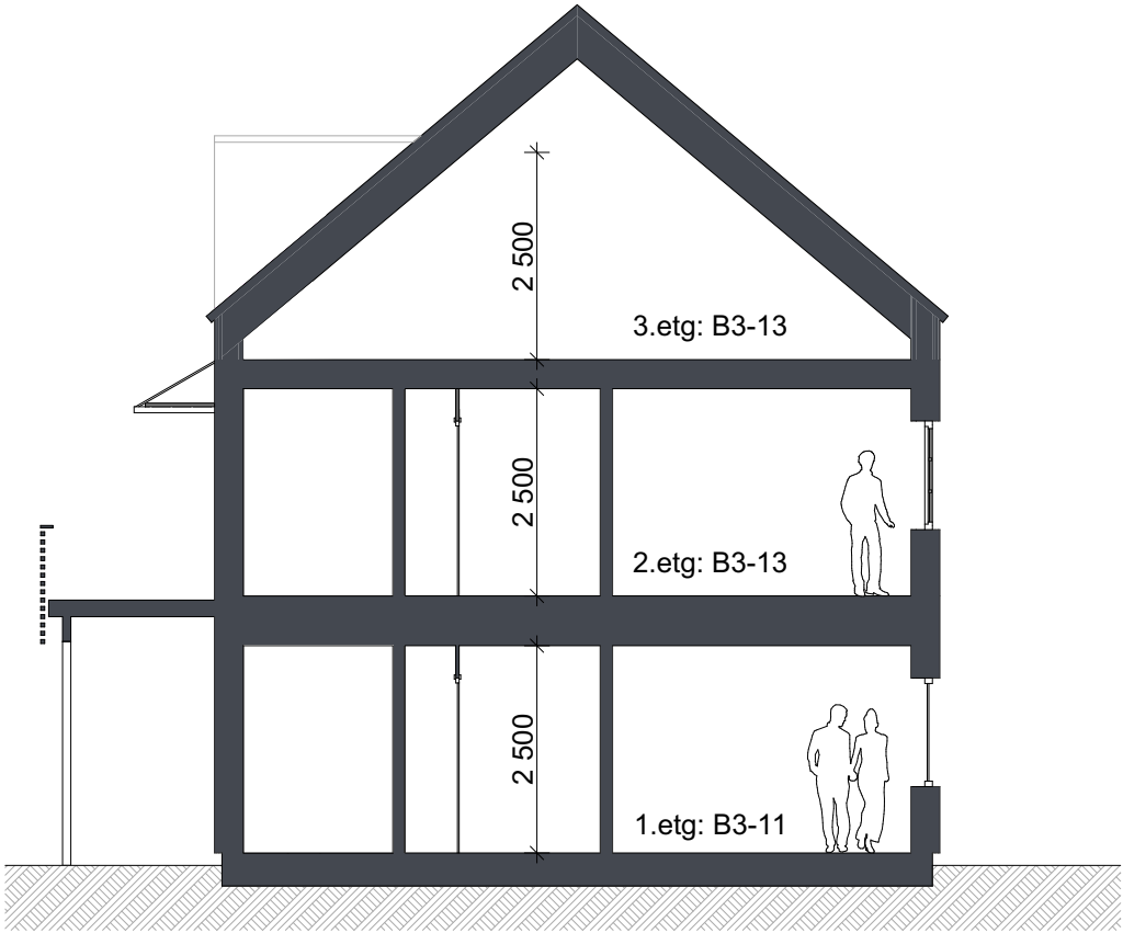
Snitt B3-11 og B3-13
