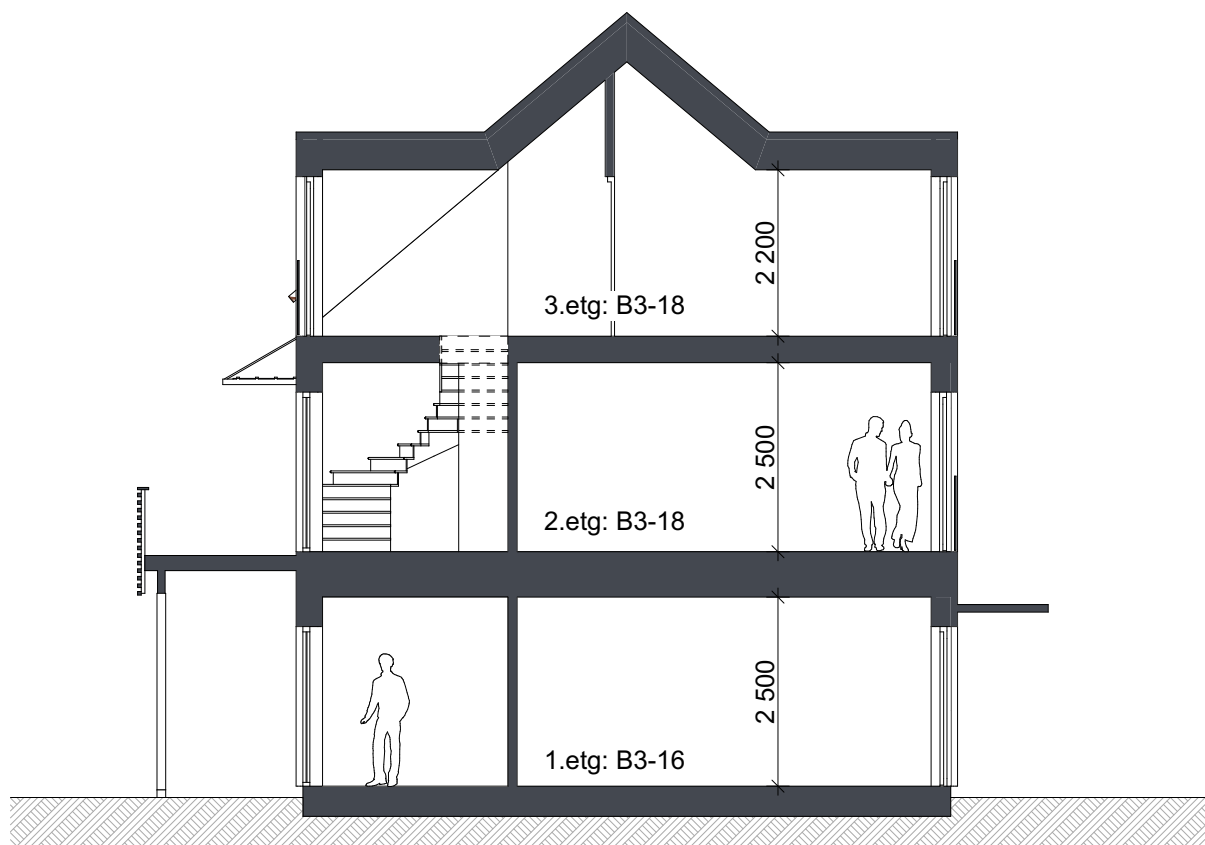
Snitt B3-16 og B3-18
